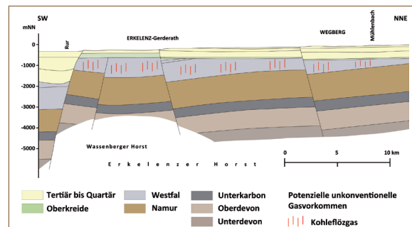
Abb. 4-2: Schematisches geologisches Profil Geosystem Südlicher Niederrhein
