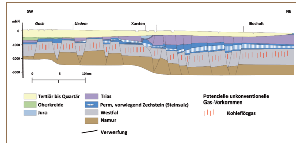
Abb. 4-1: Schematisches geologisches Profil Geosystem Nördlicher Niederrhein
