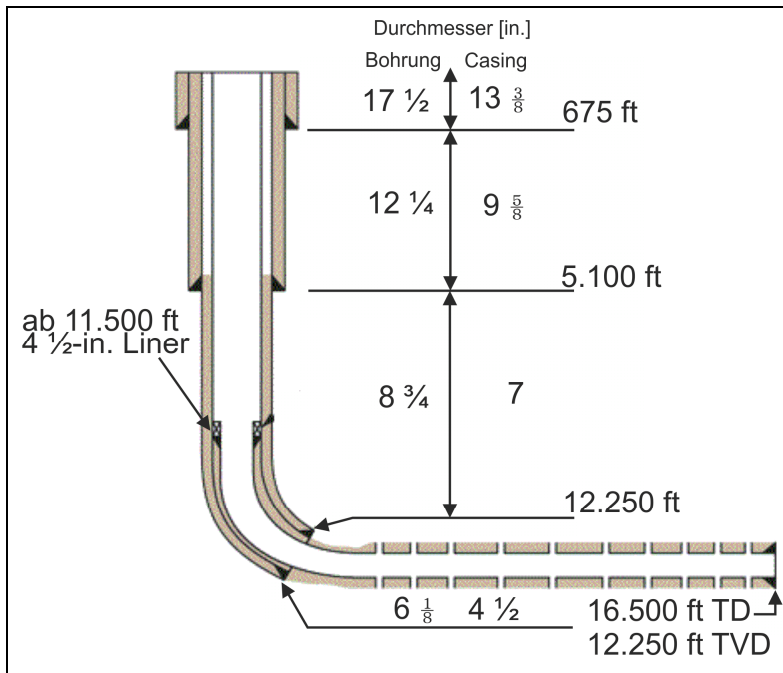
Abb. A 19: Beispielhaftes Verrohrungsschema einer Horizontalbohrung (unmaßstäblich). TD: Länge der Bohrung gemessen vom Bohrersatzpunkt (total depth); TVD: Vertikaler Abstand des Bohrlochtiefsten zum Bohrersatzpunkt (true vertical depth); Maßangaben: 1 ft = 0,3048 m; 1 in. = 2,54 cm (nach Rohwer et al. 2006)
